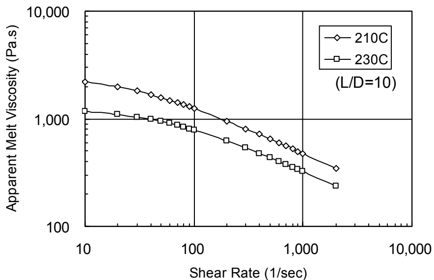
Fig. 1 Melt Viscosity of SoarnoL™ D2908
