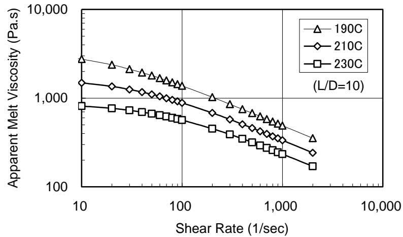
Fig. 1 Melt Viscosity of Soarnol™ A4412
