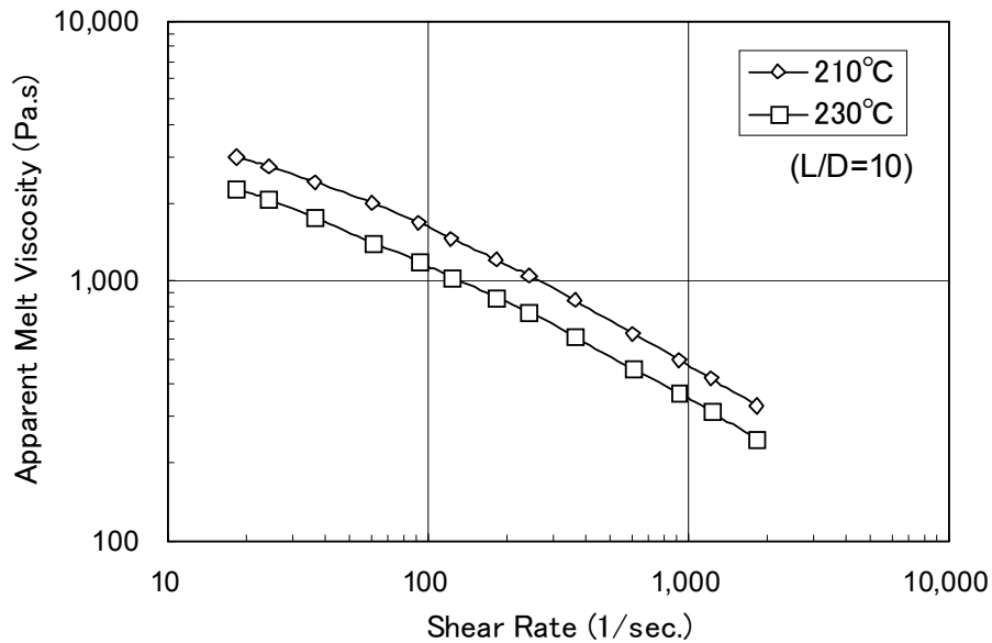
Fig. 1 Melt Viscosity of Soarnol™ BX6804B
